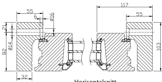
Horizontalsnitt
