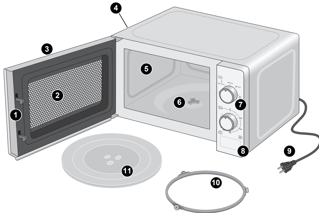
Abb. 1: Ovnens dele
