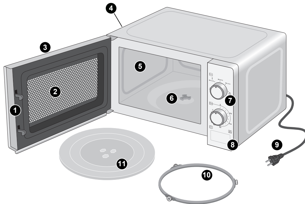
Abb. 1: Apparats delar
