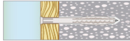
3. Montage i Lättbetong
