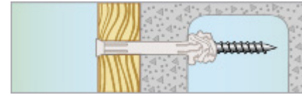
4. Montage i Hålsten
