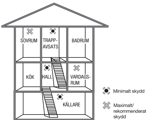
FIGUR 2. Flervånings bostad
